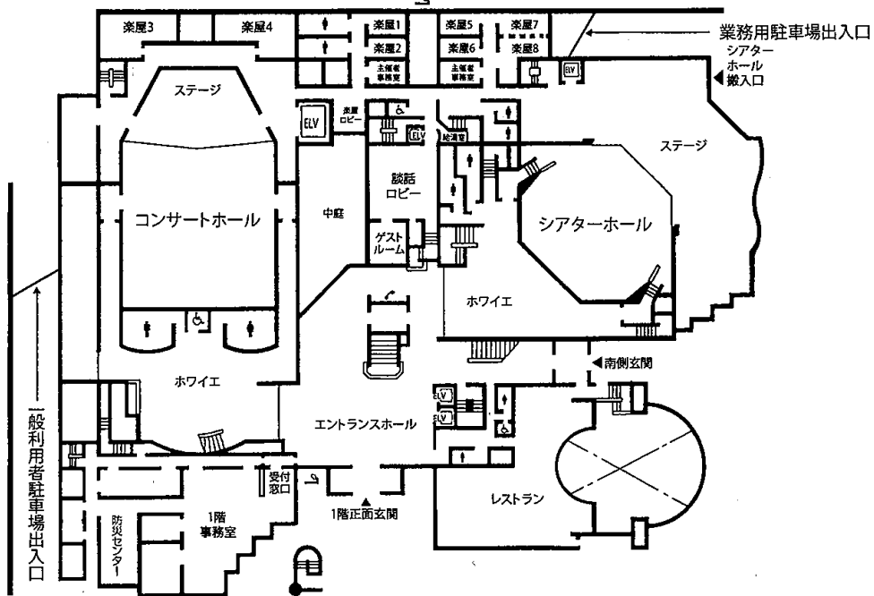
1階平面図
