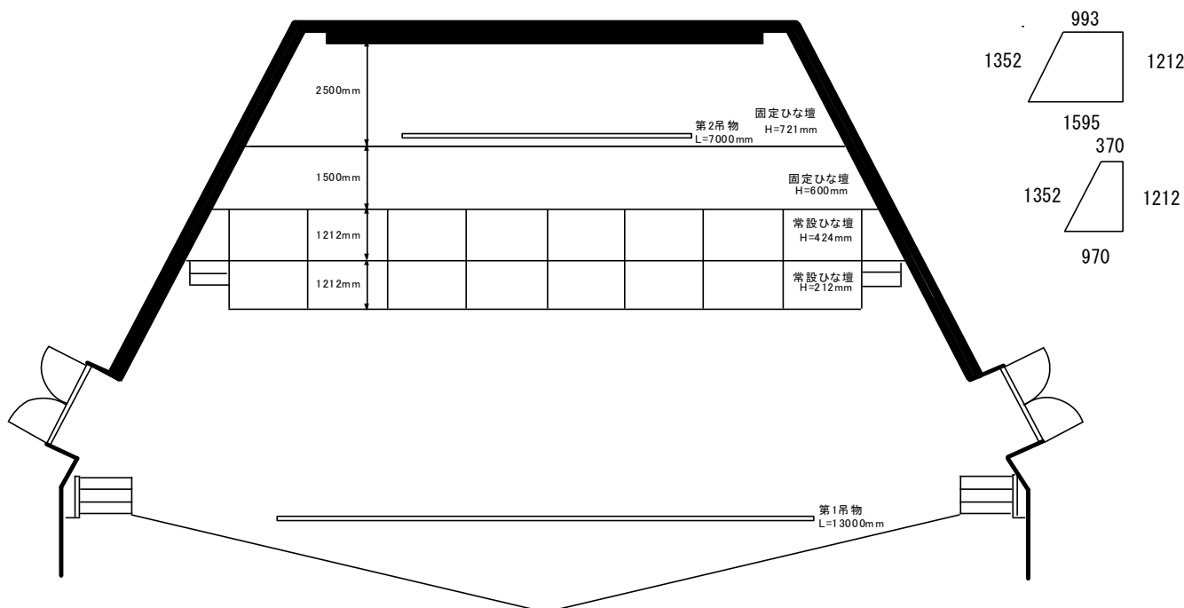
[変形平台(大・小)のサイズ]
